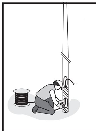
3. Zasunutí přívodního kabelu do sloupu
