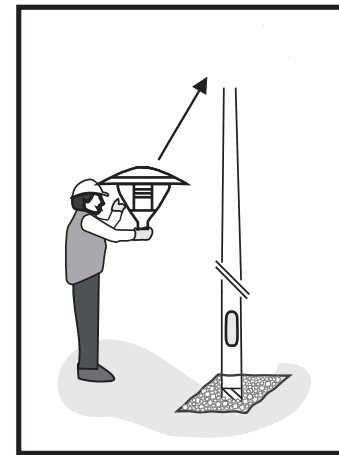
8. Namontování svítidla na sloup
