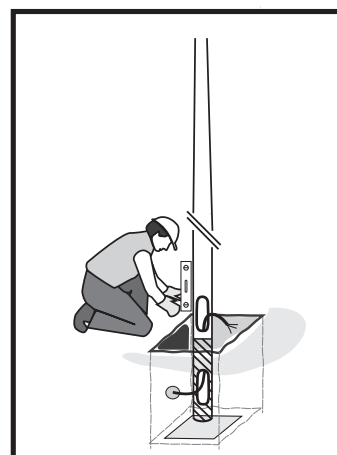
6. Osazení sloupu do vodováhy
