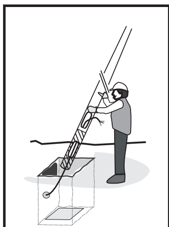
5. Vložení sloupu do výkopu
