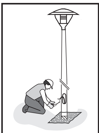
9. Zapojení elektročáští a zavření revizních dvířek
