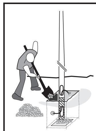
7. Zасыпání výkopu zeminou smíchanou s pískem
